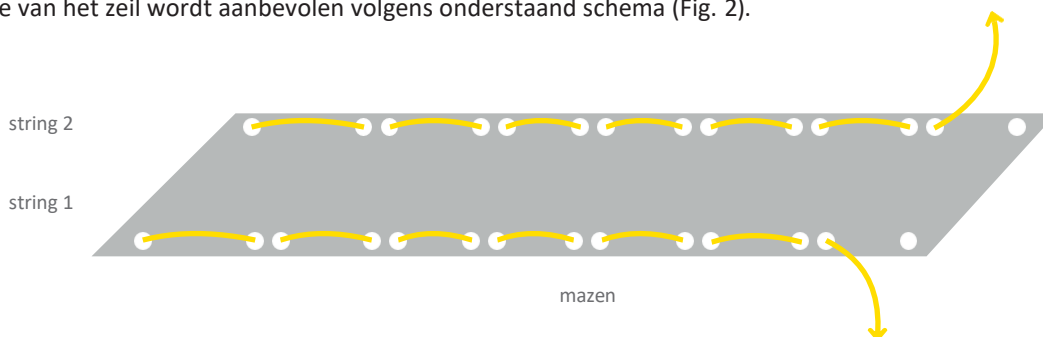
Afbeelding 2: Voorgestelde montagemethode voor het HDPE-schuifzeil
