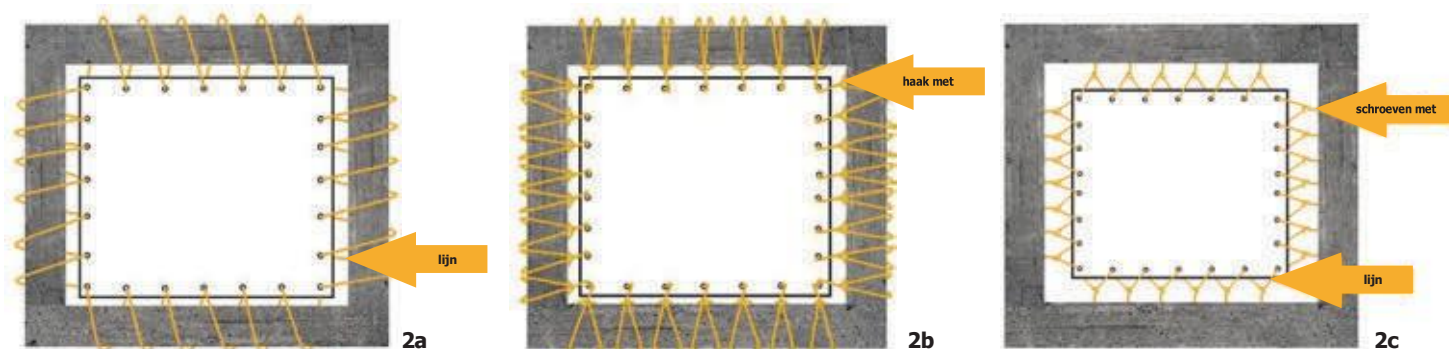
Afbeelding 2: Voorgestelde installatie van het zeildak - bovenaanzicht
