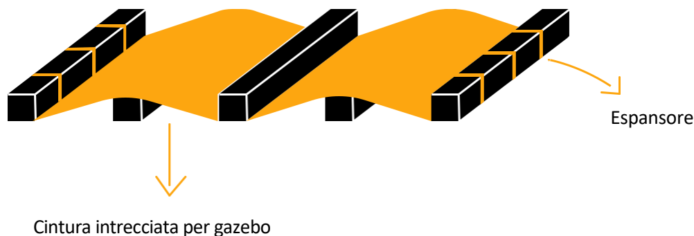
Figura 2: Proposta di installazione delle cinghie.
